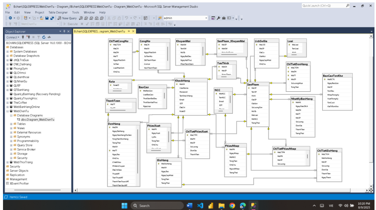
Hình 2.5 Sơ đồ diagram của website bán lẻ điện tử
